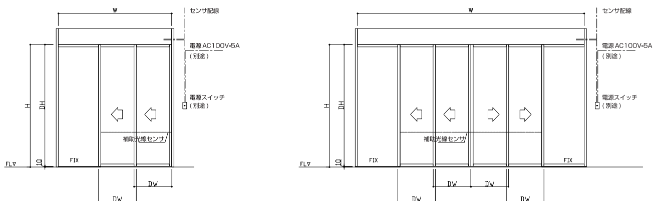
【点検口側観図】
